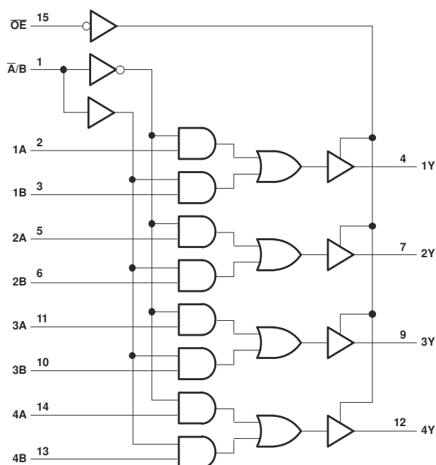
論理図 (正論理)
