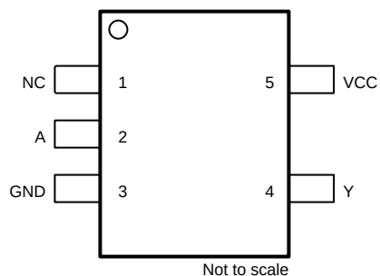
図 4-1. SN74LVC1G16-Q1 DBV パッケージ、5 ピン SOT-23 (上面図)
