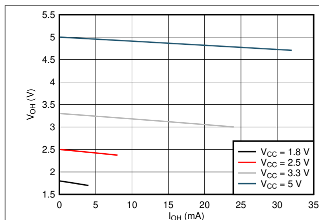
図 5-1. 典型的な V_{OH} と I_{OH} との関係 - 25°C
