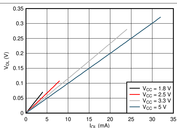
図 5-2. 典型的な V_{OL} と I_{OL} との関係 - 25°C
