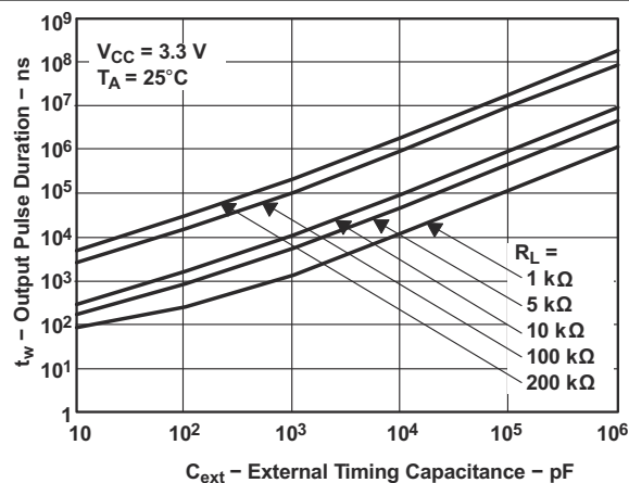
図 5-4. 出力パルス幅 と外部タイミング容量との関係
