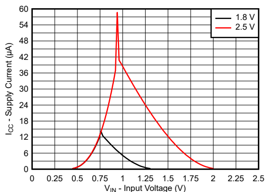
図 5-2. 入力電圧に対する電源電流、1.8V および 2.5V 電源
