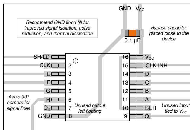
図 8-3. PW パッケージに封止した SN74LVC165A-Q1 のレイアウト例
