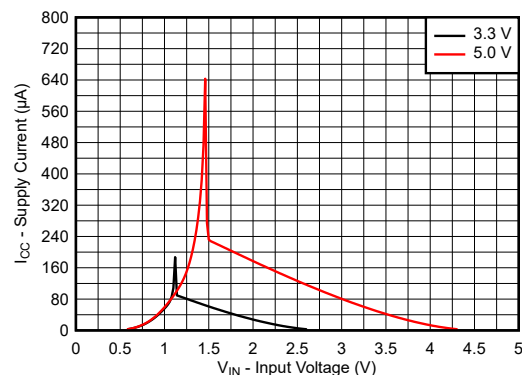
図 5-3. 入力電圧に対する電源電流、3.3V および 5.0V 電源
