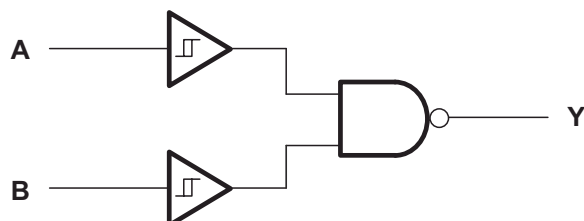
図 7-1. 各ゲートの論理図 (正論理)
