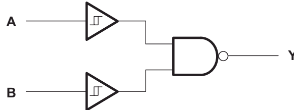
図 7-1. 各ゲートの論理図 (正論理)
