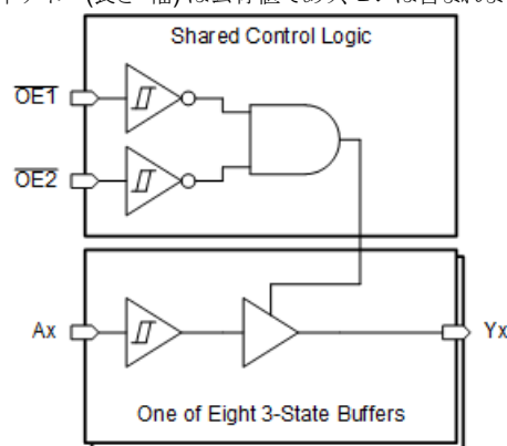
論理図 (正論理)
