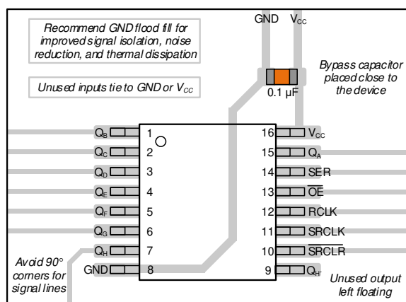
図 8-3. TSSOP の SN74LV8T596 のレイアウト例
