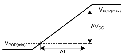
図 8-1. 既知のパワーアップ状態での電源 (V CC ) ランプ特性
