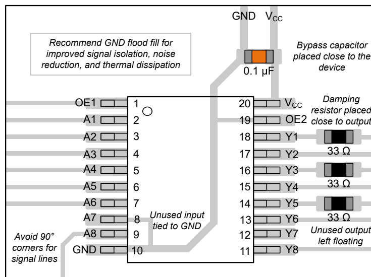
図 10-3. TSSOP の SN74LV8T541 のレイアウト例
