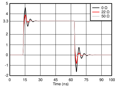
図 10-2. 異なるダンピング抵抗 ( R_d ) 値を使用してレシーバでの信号の整合性をシミュレート
