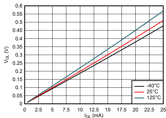
図 5-6. Low 状態における出力電圧と電流の関係、3.3V 電源
