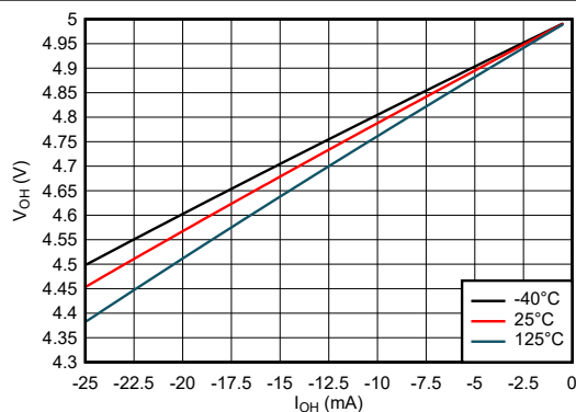
図 5-3. High 状態における出力電圧と電流の関係、5V 電源
