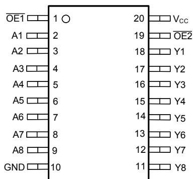
図 4-1. PW および DGS パッケージ、20 ピン TSSOP (上面図) 図 4-2. RKS パッケージ、20 ピン VQFN (透過上面図)
