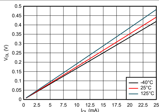
図 5-4. Low 状態における出力電圧と電流の関係、5V 電源
