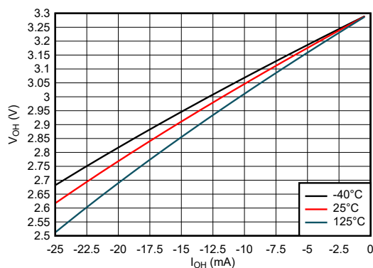
図 5-5. High 状態における出力電圧と電流の関係、3.3V 電源
