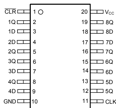
図 4-2. SN74LV8T273-Q1 PW、DGS パッケージ (上面図)
