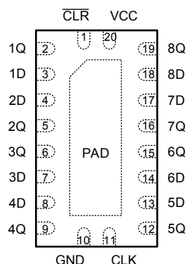
図 4-1. SN74LV8T273-Q1 RKS または RGY パッケージ
