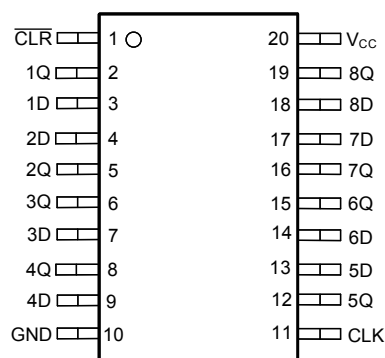
図 4-2. SN74LV8T273 PW、DGS パッケージ (上面図)
