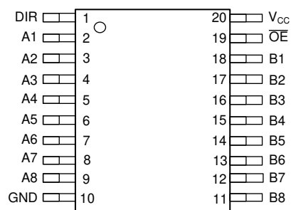
図 5-2. DGS or PW Package, 20-Pin VSSOP or TSSOP (Top View)
