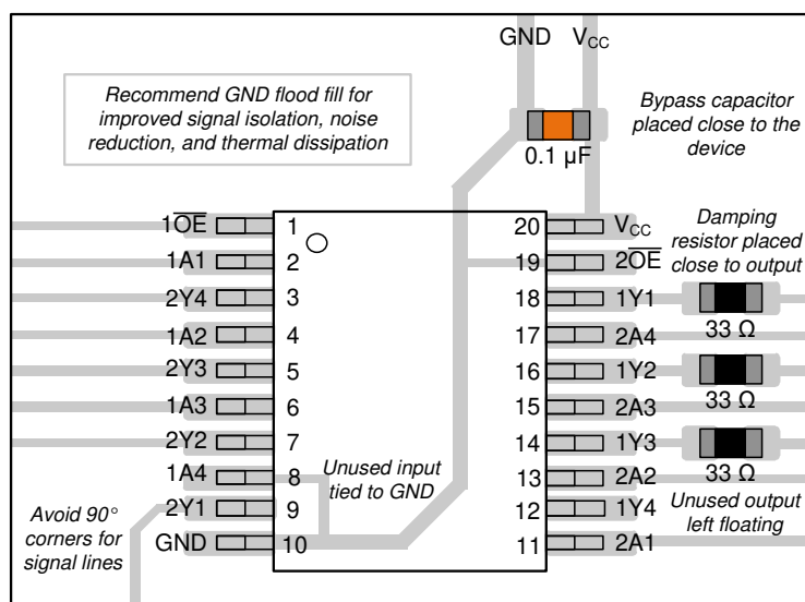
図 10-3. TSSOP の SN74LV8T244-EP のレイアウト例
