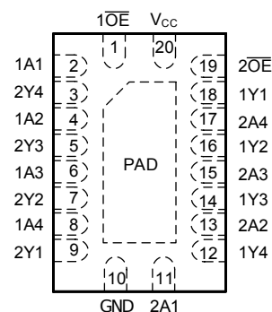
図 4-2. SN74LV8T240-Q1 RKS パッケージ、20 ピン TSSOP (上面図)
