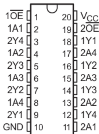
図 4-1. SN74LV8T240-Q1 PW または DGS パッケージ、20 ピン TSSOP または VSSOP (上面図)
