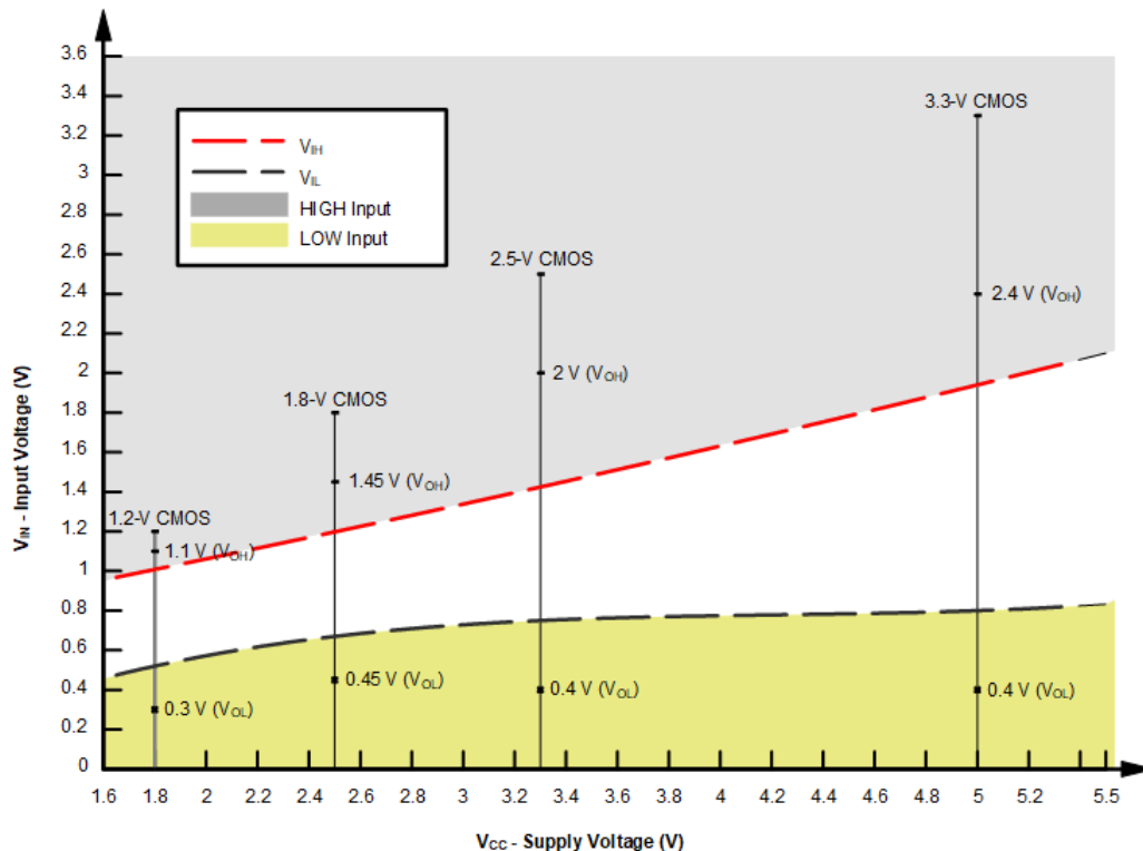
図 7-2. LVxT の 電圧レベル
