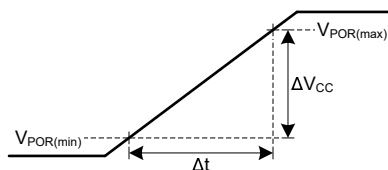
図 7-3. 既知のパワーアップ状態での電源 ( V_{CC} ) ランプ特性
