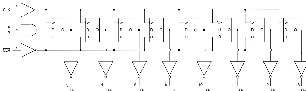
論理図 (正論理)
