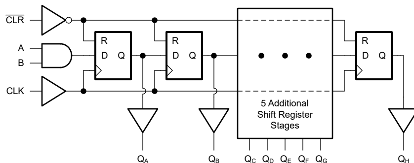
概略論理図 (正論理)
