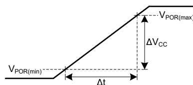
図 7-1. 既知のパワーアップ状態での電源 ( V_{CC} ) ランプ特性
