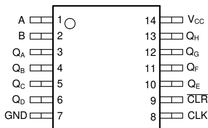
図 4-1. PW パッケージ、14 ピン TSSOP (上面図)
