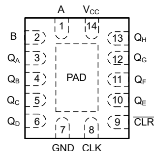
図 4-2. BQA パッケージ、14 ピン WQFN (透過上面図)
