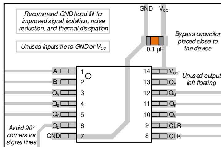
図 8-3. TSSOP の SN74LV8T164 のレイアウト例
