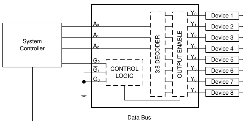
図 8-1. マルチプレクサによる出力拡張
