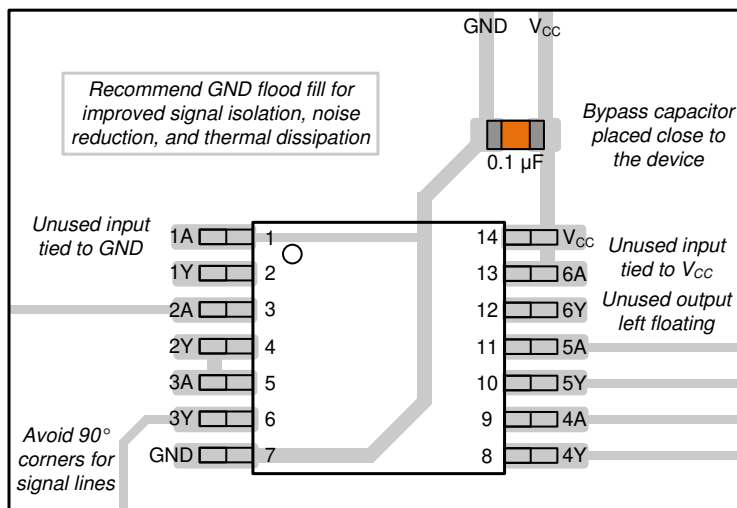
図 8-3. SN74LV6T14-EP のレイアウト例
