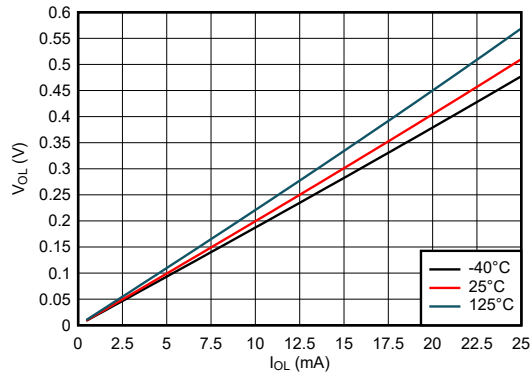
図 5-9. Low 状態における出力電圧と電流との関係、1.8V 電源
