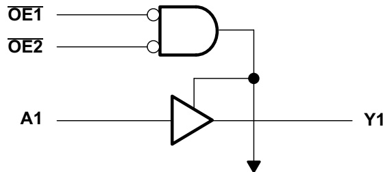
概略回路図
