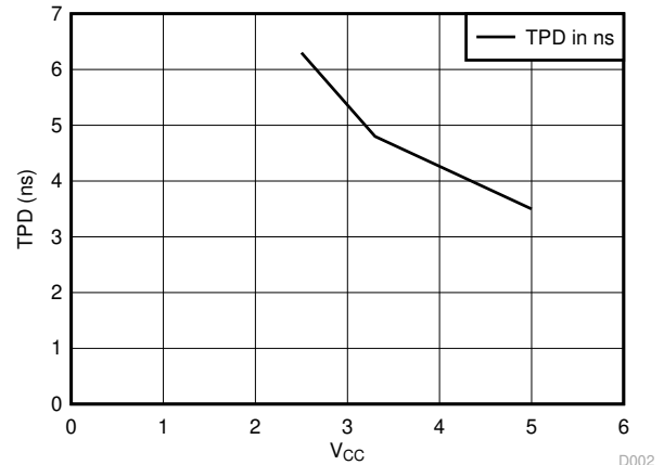
図 6-8. 25°Cでの TPD と V_{CC} との関係
