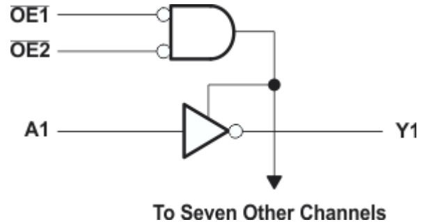
図 3-1. 簡略回路図
