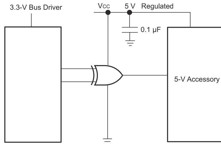
図 8-1. 代表的なアプリケーション回路図
