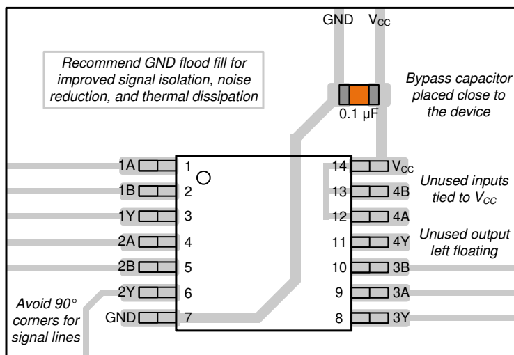
図 8-3. レイアウト例 : SN74LV4T86-EP
