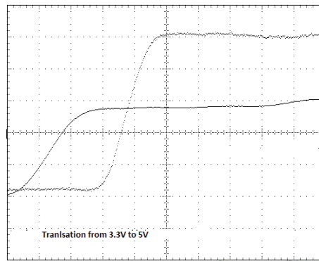
図 8-2. 昇圧変換
