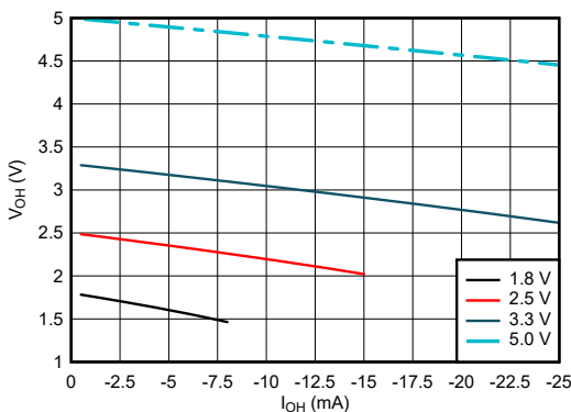
図 6-3. High 状態における出力電圧と電流との関係
