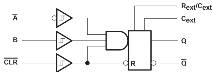
図 6-1. 各マルチバイブレータの論理図 (正論理)
