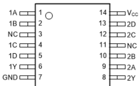
図 3-1. SN74LV20A D、DB、DGV、NS、PW パッケージ、14 ピン SOIC、SSOP、TVSOP、SOP、TSSOP (上面図)
