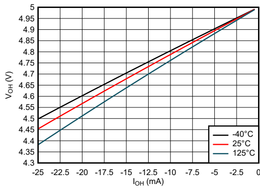
図 5-6. High 状態における出力電圧と電流との関係、 5V 電源
