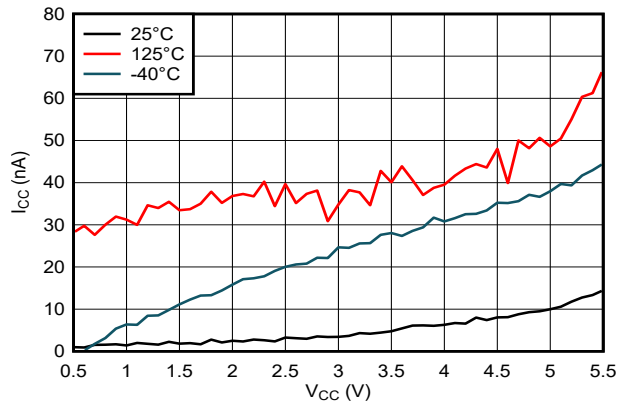
図 5-3. 電源電圧間の電源電流
