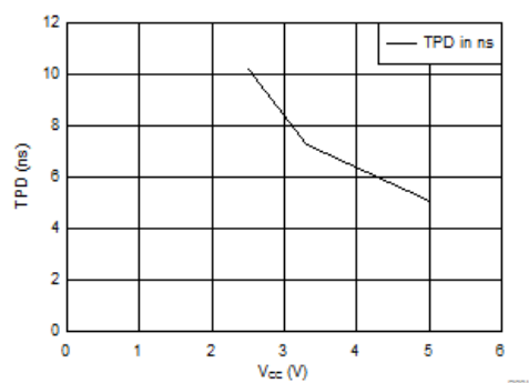
図 6-1. TPD と V_{CC} との関係
