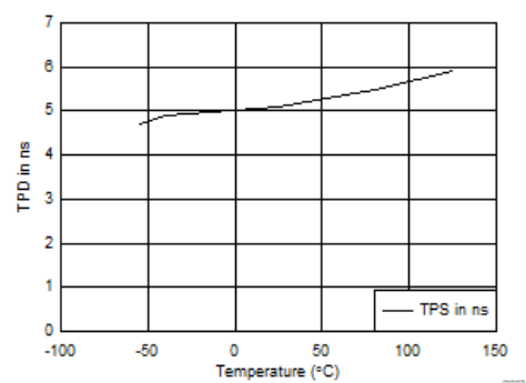
図 6-2. TPD と温度との関係
