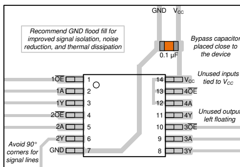
图 11-1. Example layout for the SN74HCS125-Q1
