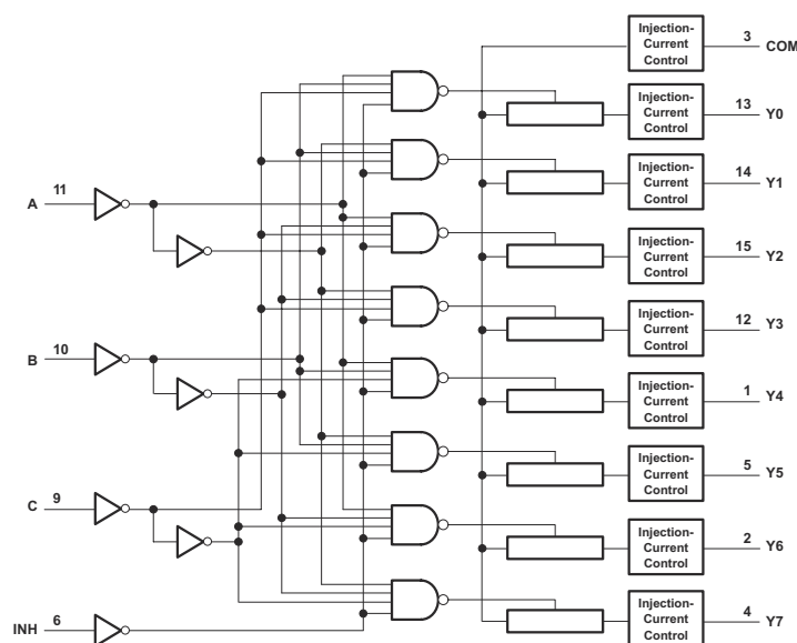
論理図 (正論理)
