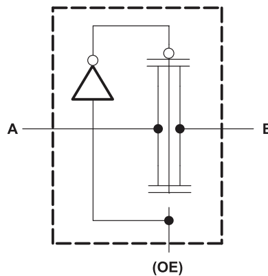
図 6. Simple Schematic
