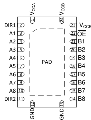
図 4-2. RHL および WRGY パッケージ、24 ピン VQFN (上面図)
