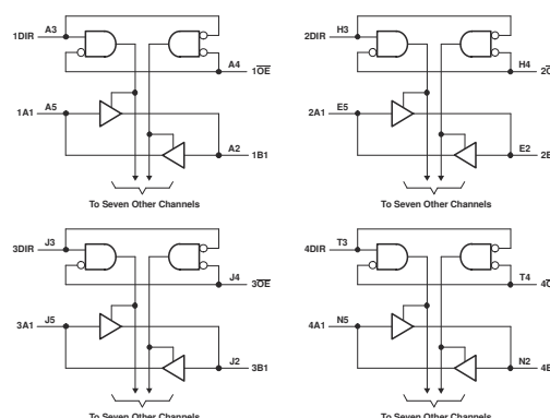
図 3-1. ロジック図
