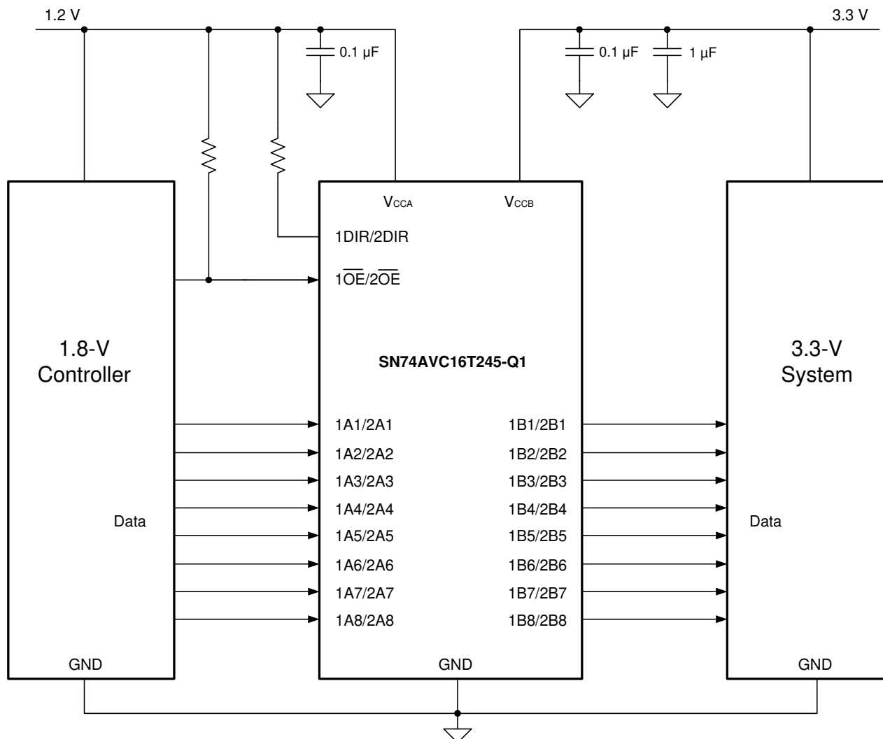
図 9-1. 代表的なアプリケーション回路図
