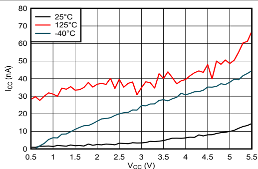
図 5-2. 電源電流と電源電圧との関係
