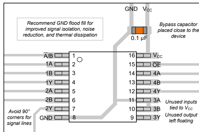
図 8-3. SN74AHCT257 のレイアウト例
