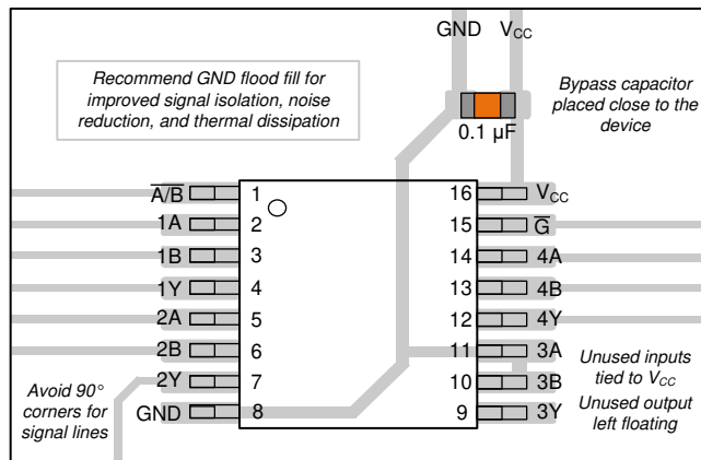
図 8-3. SN74AHCT157-Q1 のレイアウト例
