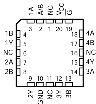
NC – No internal connection 図 3-2. SN54AHCT157 FK パッケージ (上面図)
