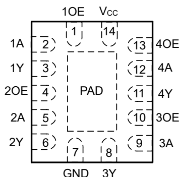
図 4-1. BQA パッケージ、14 ピン WQFN (上面図)
