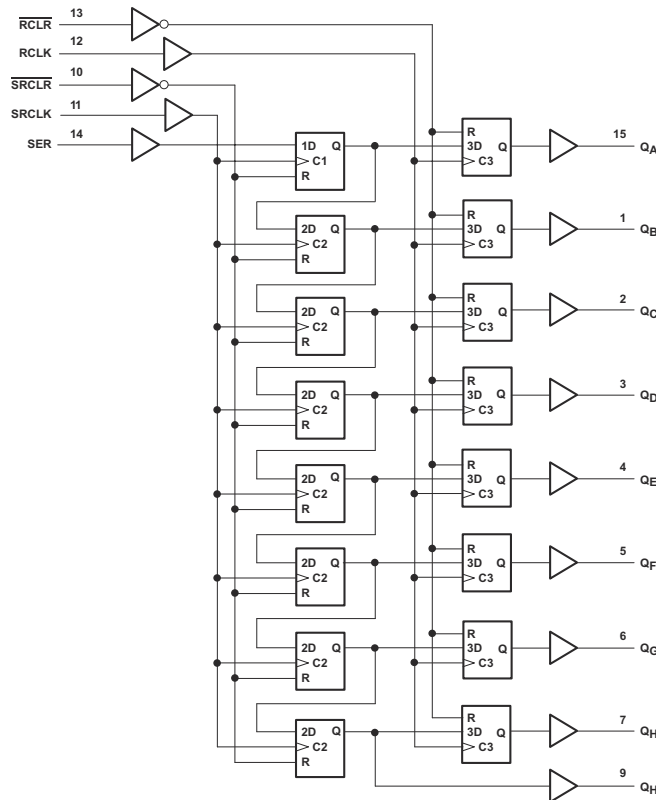
概略回路図
