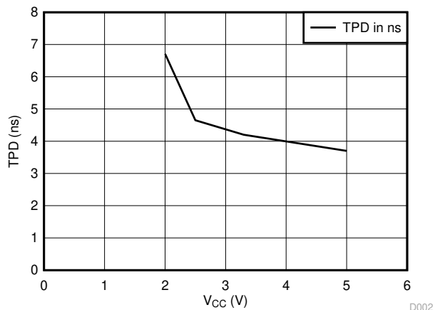
図 5-3. TPD vs V CC
