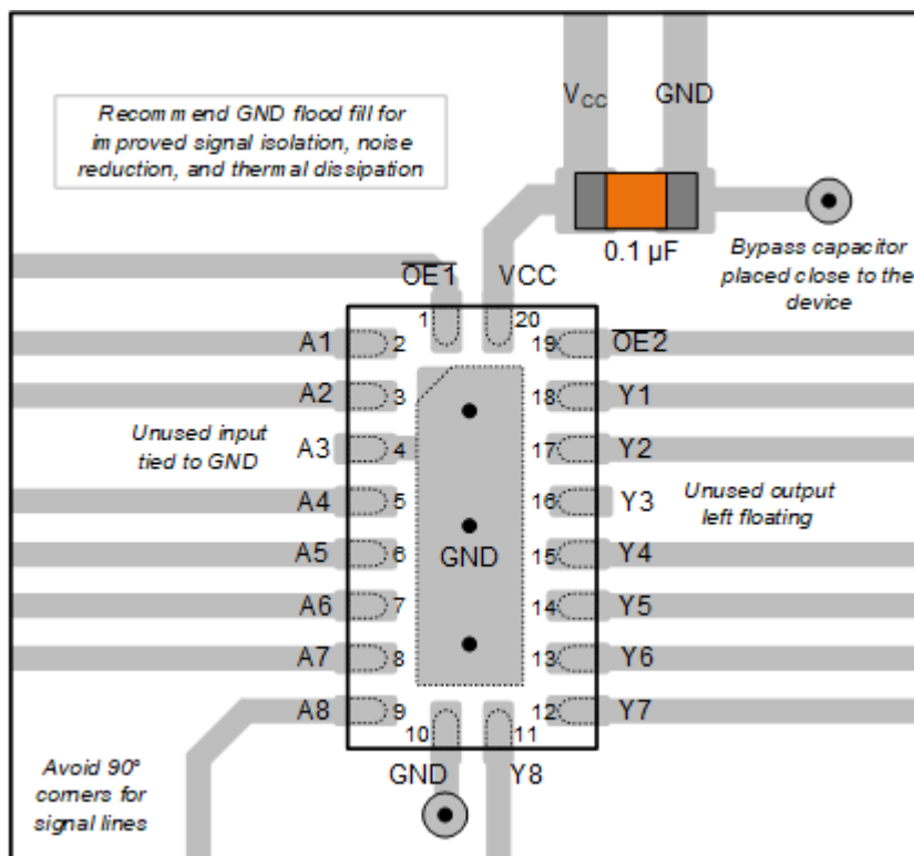
図 8-1. Layout Diagram
