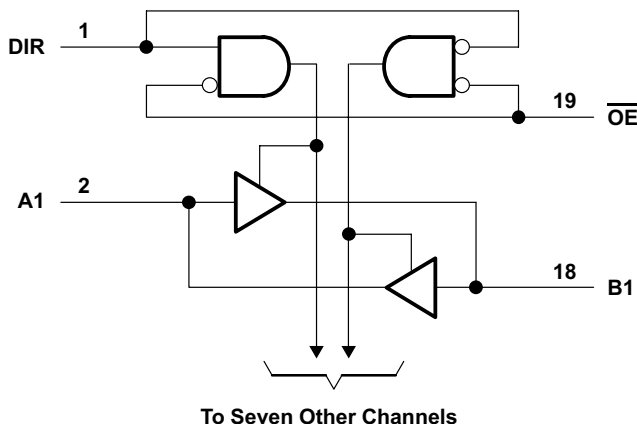
概略回路図
