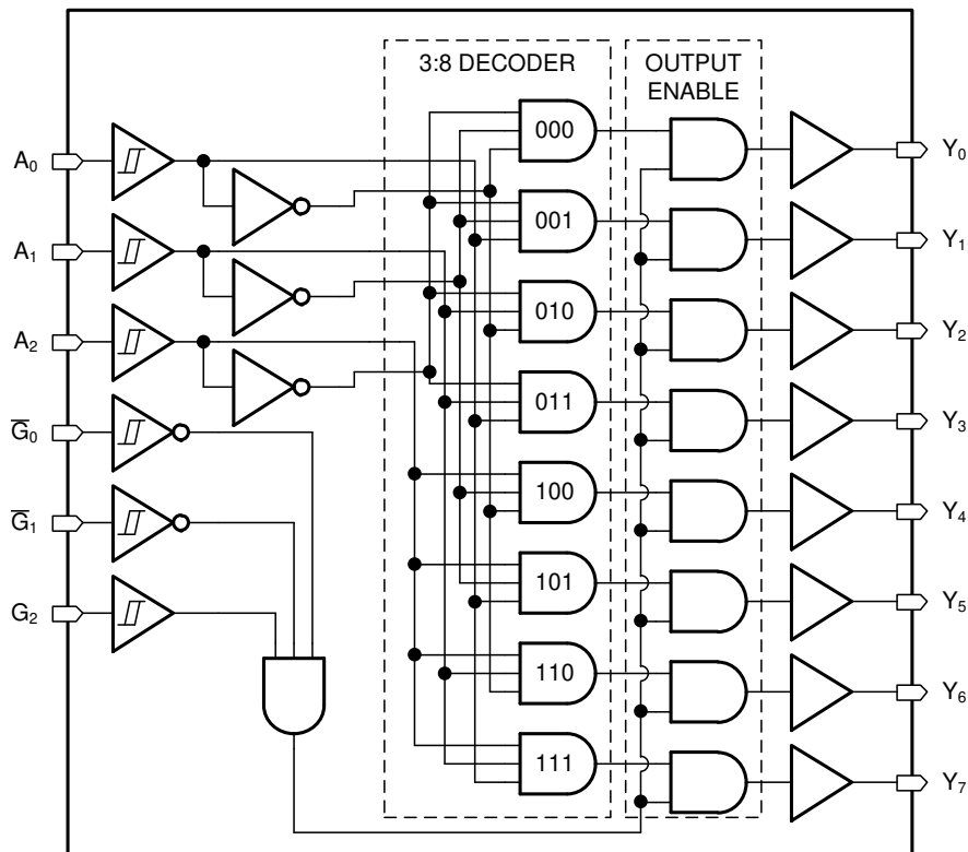
図 7-1. SN74AHC238-Q1 の論理図 (正論理)
