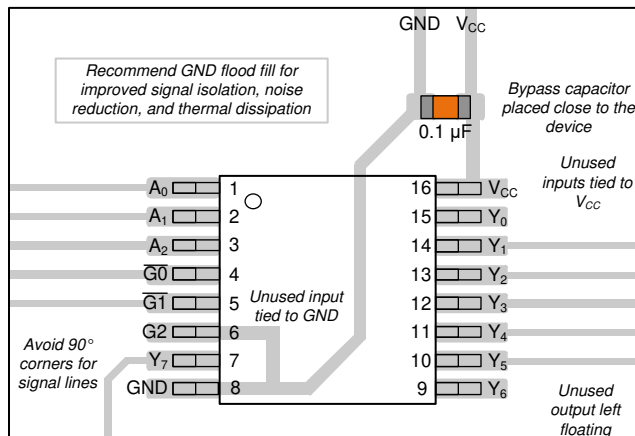
図 8-3. SN74AHC238-Q1 のレイアウト例
