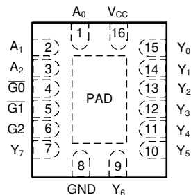
図 4-2. BQB パッケージ、 16 ピン WQFN (透視上面図)
