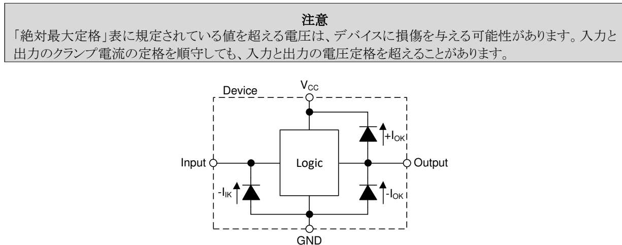
図 7-2. 各入力と出力に対するクランプ ダイオードの電気的配置
