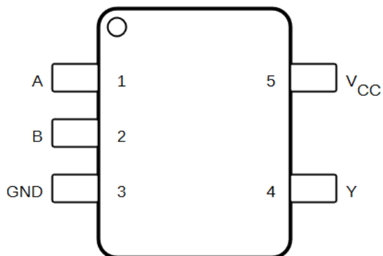
図 4-1. DCK パッケージ、5 ピン SC70 (上面図)
