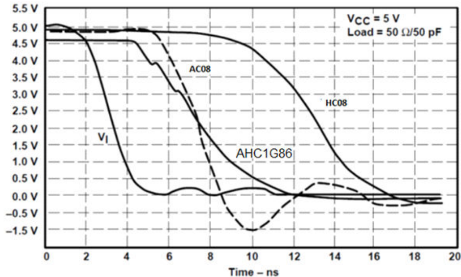
図 8-2. スイッチング特性の比較
