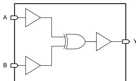
図 7-1. 排他 OR ロジック
