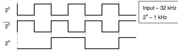
図 9-2. アプリケーションのタイミング図
