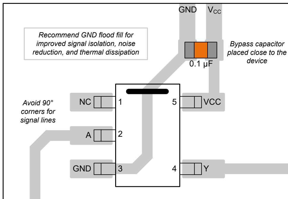
図 9-3. SN74AHC1G14-Q1 のレイアウト例
