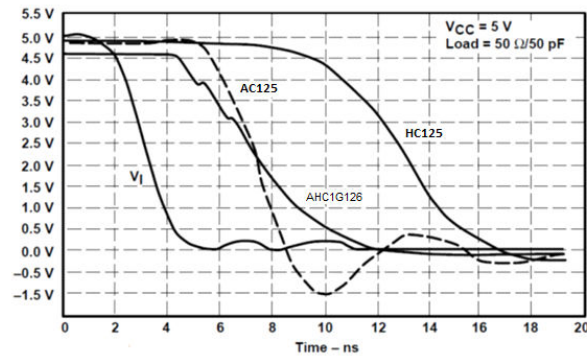
図 8-2. 出力ターンオフ波形
